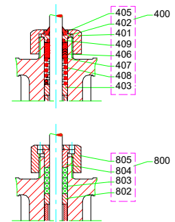
DN 15-65, PN 16-40
