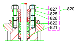
DN 80-100, PN 16-40
